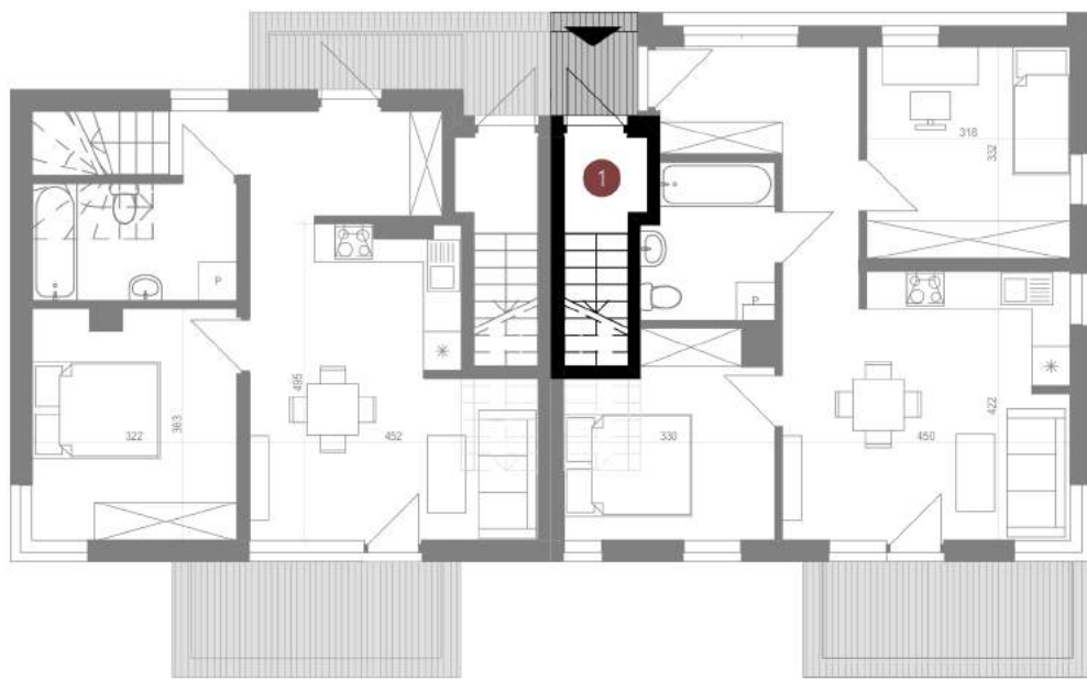
RZUT PARTERU
